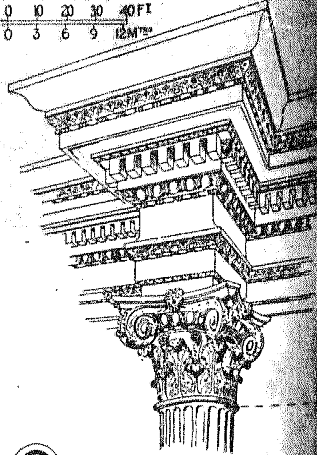
G CAPITAL & ENTABLATURE
